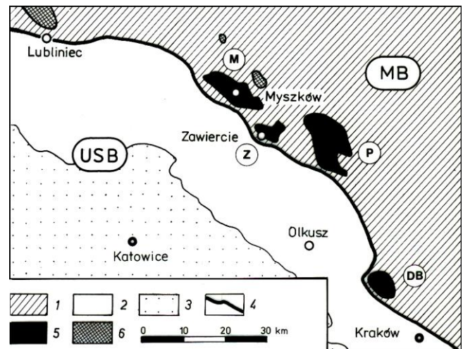
Rys. 2. Położenie Olkusza – z wystąpieniami tzw. „zlepieńca parczewskiego” – na tle strefy granicznej bloków górnośląskiego i małopolskiego (ŻABA, 1995, 1999):
