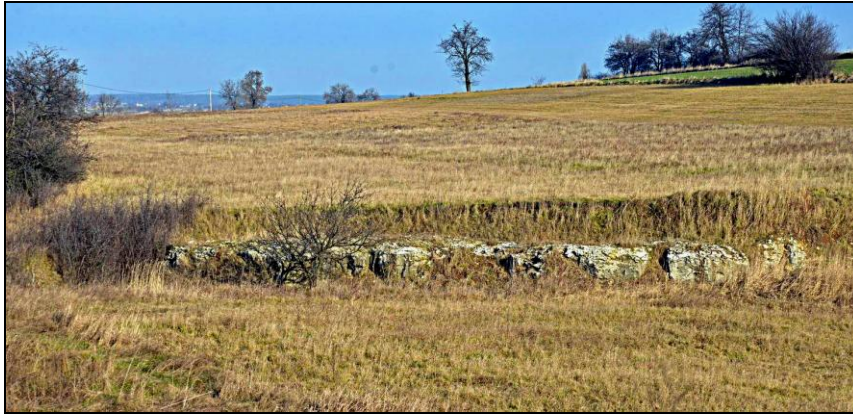
Fot. 3. Wychodnia wapieni woźnickich w miejscowości Wojsławice (fot. J. Nita) Photo.3. Outcrop of limestone in Wojsławice (phot. by J. Nita)
